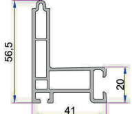
Sineklik Ray Profili P.A.232.5802.600.0.00.19
