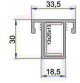
Sürme Sineklik Orta Kayıt Profili P.A.242.3200.600.0.00.01
