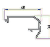
Alm. Kasa Kanal Kapama Profili AD 16 - 013
