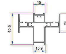
Alm. Kulaklı Çift Kanat Adaptörü Profil YENİ Yapılacak
