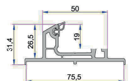
Çift Ray Adaptör Profili P.A.232.5800.600.0.00.19
