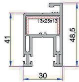
Sürme Sineklik Kanat Profili P.A.242.2305.600.0.00.01
