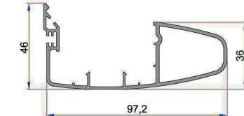
Alm. Kanat Arka Kapama Griyalı Profili 16028.601.5.2.0.9016
