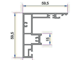
Üç Bölmeli Sürme Alm. Orta Kayıt Profili Profil YENİ Yapılacak
