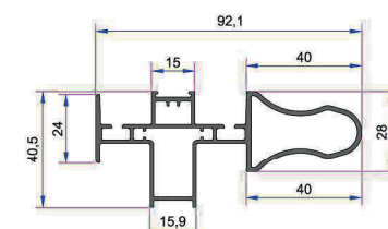
Alm. Griyalı Çift Kanat Adaptörü Profil YENİ Yapılacak
