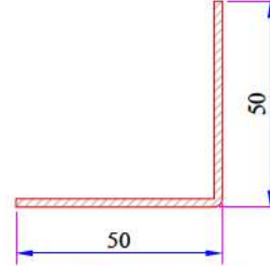
90° Köşe Profili Destek Sacı 34022-12302
