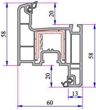
Kanat Profili 624.2000
