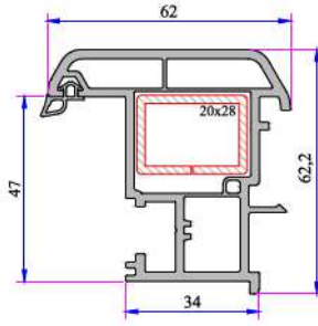
Hareketli Orta Kayıt Profili 632.3104
