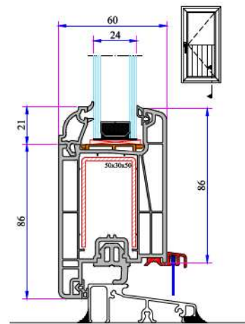
Alüminyum Eşikli Kasa - Kapı Kanat Profil Montajı
