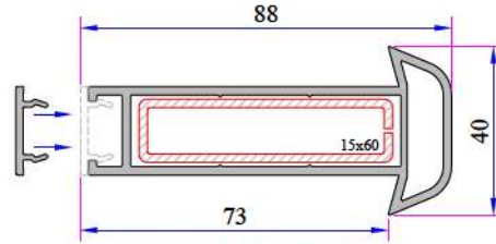
Universal Kalın Bağ Profili 058.5000
