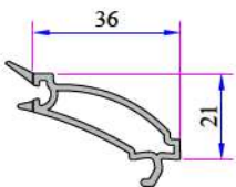
Tek Cam Çıtası 4-6 mm 101.4002
