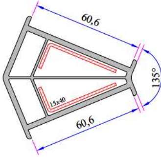
135° Köşe Profili 060.5102
