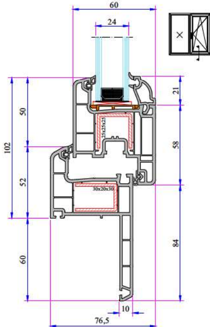
Pervazlı Kasa (60mm) - Kanat Profil Montaj
