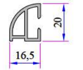
Damlalık Profili 900.6307
