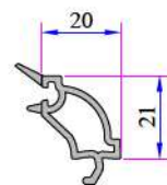
Çift Cam Çıtası 20 mm 101.4102
