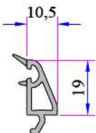
Üçlü Cam Çıtası 30 mm 332.4100
