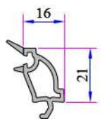
Çift Cam Çıtası 24 mm 101.4202
