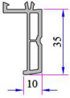
Kasa Yükseltme Profili (35mm) 099.5523
