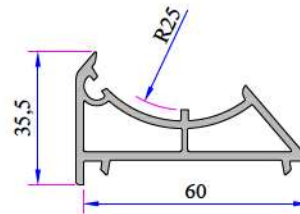
Açılı Dönüş Adaptör Profili 060.5104
