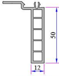
Kasa Yükseltme Profili (50mm) 099.5524
