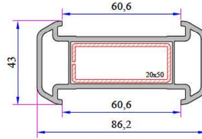
Kalın Bağ Profili 060.5000
