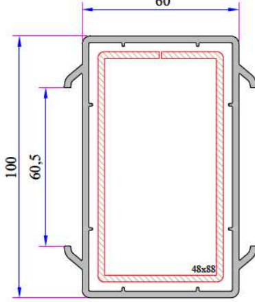
60x100 Tırnaklı Kutu Profili 060.5203
