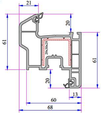
Damlalıklı Kanat Profili 632.2200
