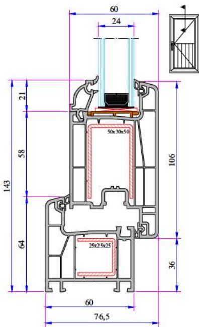
Kasa - Dışa Açılım Kapı Kanat Profil Montajı
