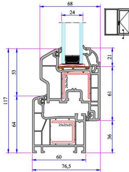
Kasa - Damlalıklı Kanat Profil Montajı
