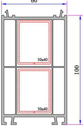
60x100 Kasa Yükseltme Profili 900.5303
