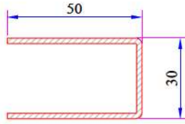
Kapı Kanat - Dışa Açılım Kapı Kanat Destek Sacı 34022-12013
