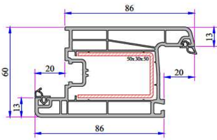
Kapı Kanat Profili 624.2100
