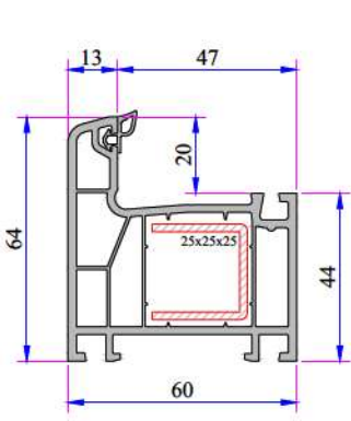
Kasa Profili 624.1000
