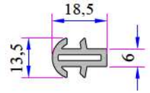
Kısa Bağ Profili 099.5003
