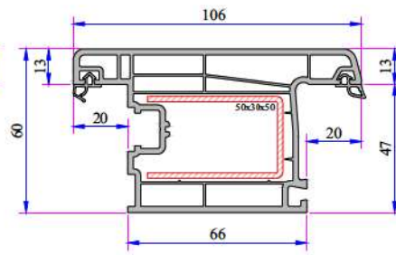
Dışa Açılım Kapı Kanat Profili 624.2101
