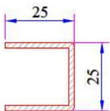
Kasa - Orta Kayıt - Kanat Destek Sacı 34022-12003
