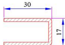
Pervazlı Kasa Destek Sacı 34022-12032
