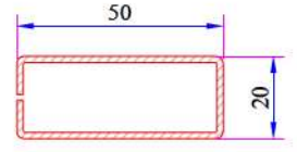
Kalın Bağ Destek Sacı 34022-12105
