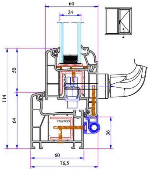
Kasa - Kanat Profil Montaj
