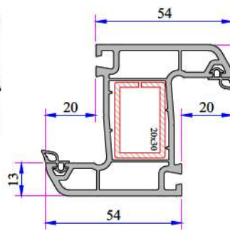
Dışa Açılım Orta Kayıt Profili 632.3005
