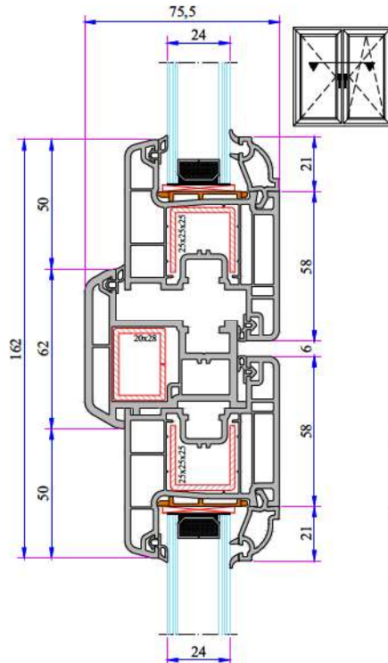
Kasa - Hareketli Orta Kayıt - Kanat Profil Montajı
