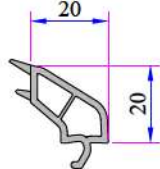
Çift Cam Çıtası 20 mm 101.4100
