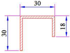
22 Akis. Dışa Açılım Kanat Destek Sacı 34022-12022
