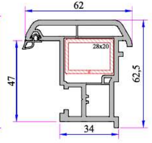
Hareketli Orta Kayıt Profili 632.3100
