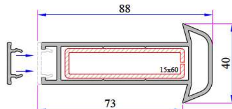
Ünliversal Kalın Bağ Profili P.A.058.5000.600.0.19
