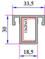
Sineklik Orta Kayıt Profili P.A.242.3200.600.0.00.03
