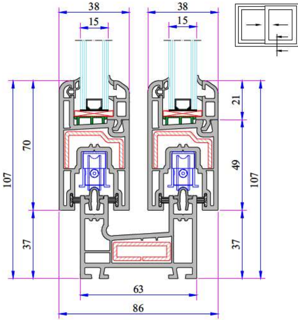
Çift Ray Sürme Kasa - Sürme Kanat Montajı
