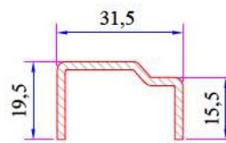
Sürme Kanat Profili Destek Sacı 34022-15026
