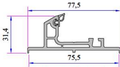
Çift Ray Adaptör Profili P.A.232.5800.600.0.BC.19
