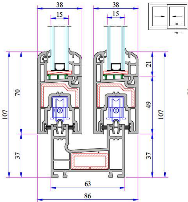
Çift Raylı Kasa (Yeni) - Sürme Kanat Montajı
