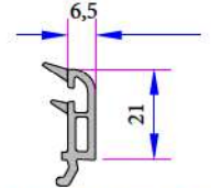
Çift Cam Çıtası 17mm P.A.532.4500.600.0.HC
