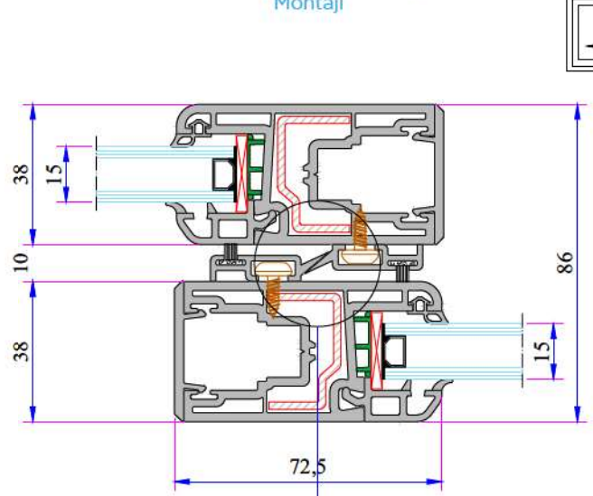
Sürme Kanat Alm. Arka Kapama Montajı
