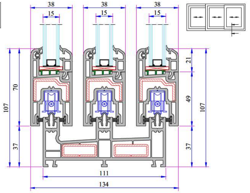
Üç Raylı Kasa - Sürme Kanat Montajı
