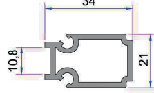
Alm. Çift Ray Adaptörü AD16-011
