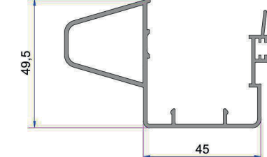
Alm. Kanat Arka Kapama Griyaj Profili Kalıp Yeni Yapılacak
