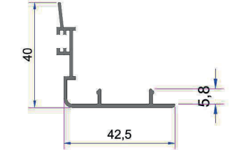
Alm. Kanat Arka Kapama Profili AD16-031
