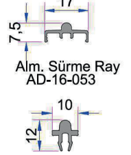
Alm. Sürme Ray AD16-053
