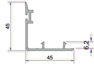
Süper Kanat Arka Kapama Profili P.A.222.5700.600.0.00.19
