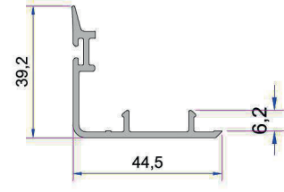
Kanat Arka Kapama Profili P.A.222.5708.600.0.00.19
