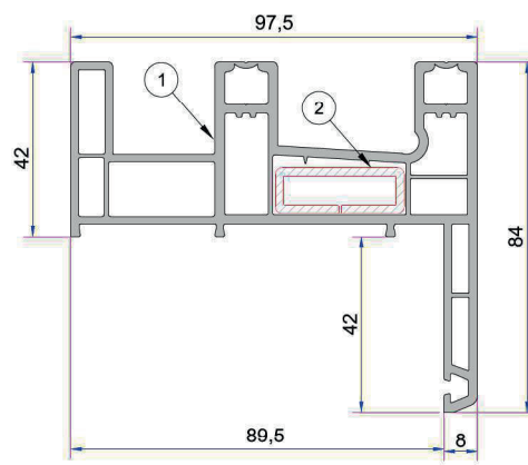
Sineklikli Sürme Kanat Kapama P.A.242.5701.650.0.00.19
