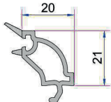
4mm Tek Cam Çıtası P.A.101.4102.600.0.HC
