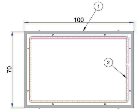
Alm. Çift Ray Adaptörü AD16-011
