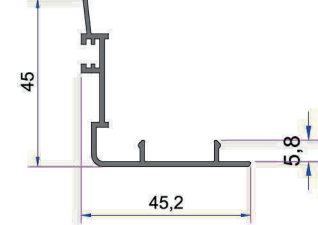
Alm. Süper Kanat Arka Kapama Profili AD16-032
